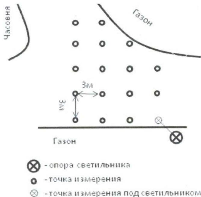
Рисунок А. Схема расположения контрольных точек проведения измерений горизонтальной освещенности.
